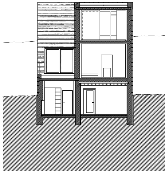
Querschnitt E-E M 1:200
