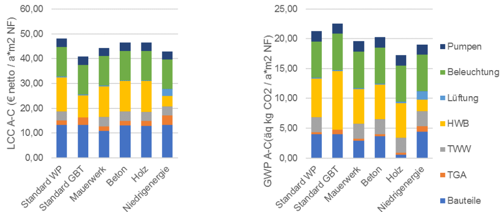
Abbildung 76: Gesamt Betrachtung LCC (links) und LCA (rechts) auf Gebäudeebene GK3 (Solitär) pro m 2 NF und a
