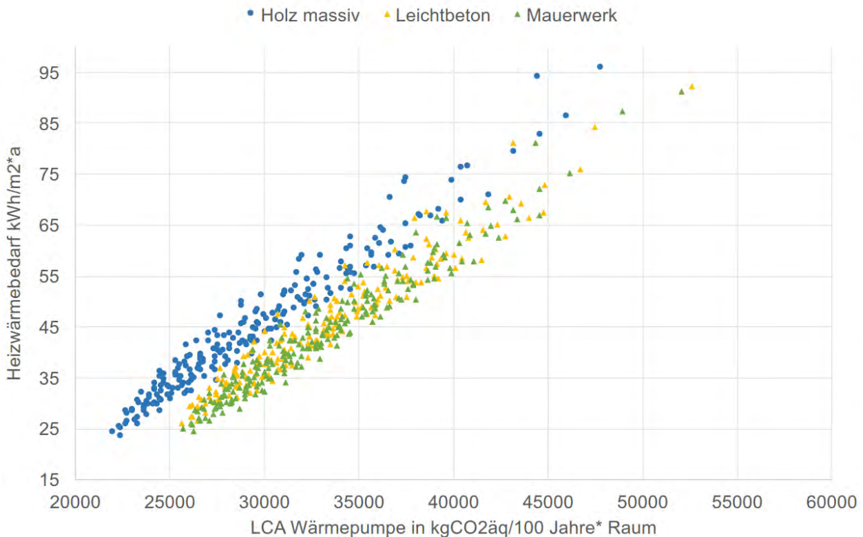
Abbildung 63: Exemplarischer Mittelraum, westorientiert, mit Darstellung des Gesamt-GWP gegenüber spezifischem Heizwärmebedarf
