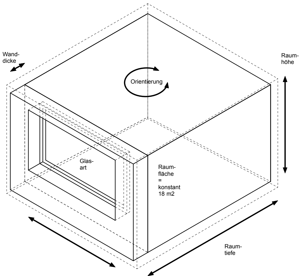
Abbildung 39: Raumgeometrie Parameter
