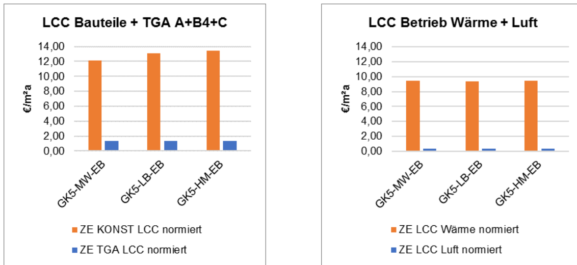
Abbildung 16: Gebäudeklasse 5 LCC Bauteile + TGA und Betrieb pro m² NF und a
