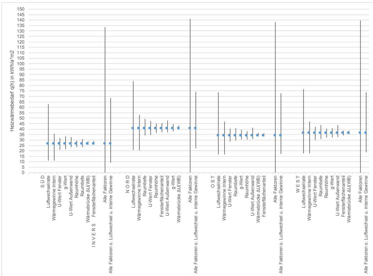
Abbildung 32: Auswirkungen der Parameterveränderungen auf den Heizwärmebedarf einzeln für die Haupthimmelsrichtungen
