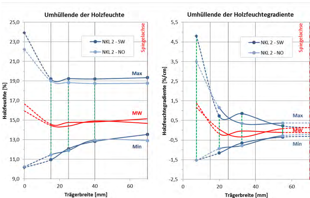
Abbildung 15: Gegenüberstellung der Umhüllenden der Holzfeuchte (links) und Holzfeuchtegradienten (rechts) über den Querschnitt des Tragwerks in NKL 2 im Süd-Westen und Nord-Osten des Gebäudes (Knorz et al. , 2016).
