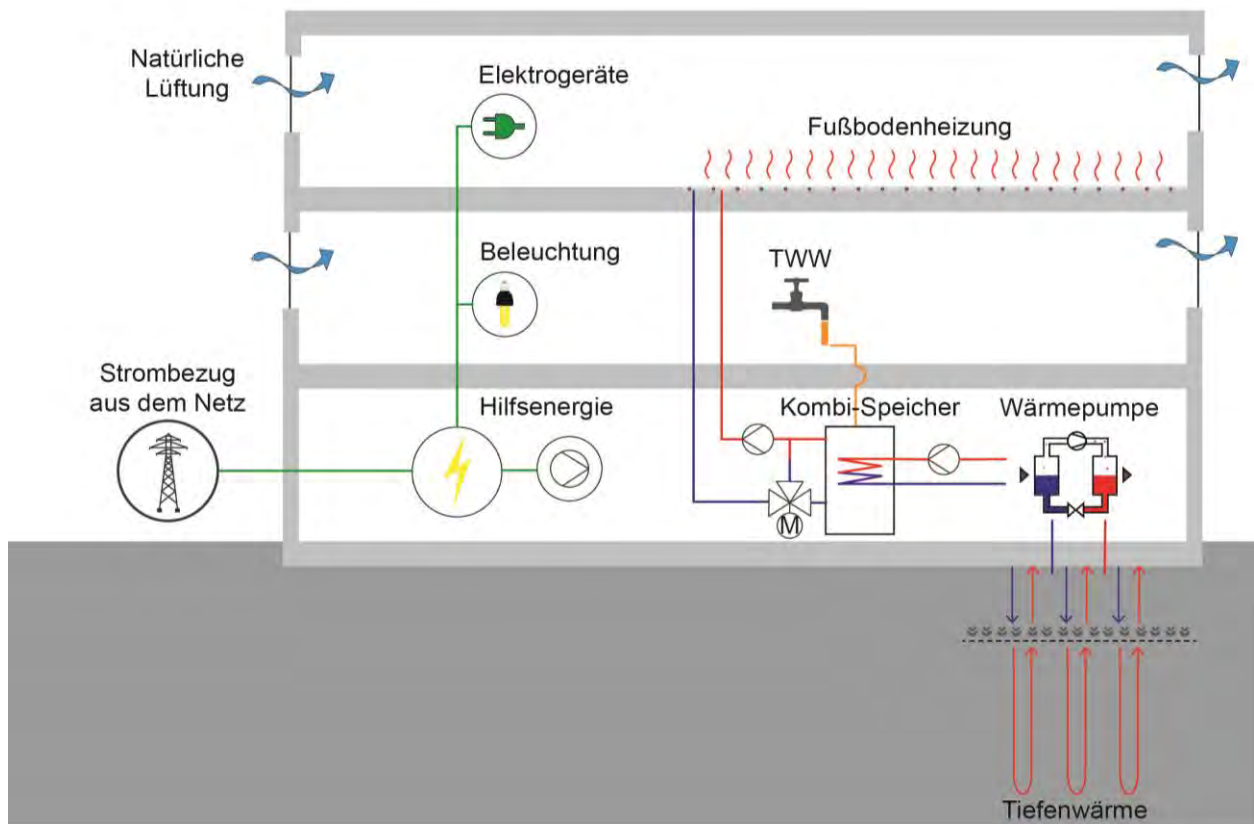
Abbildung 72: Energiekonzept Einfach Bauen
