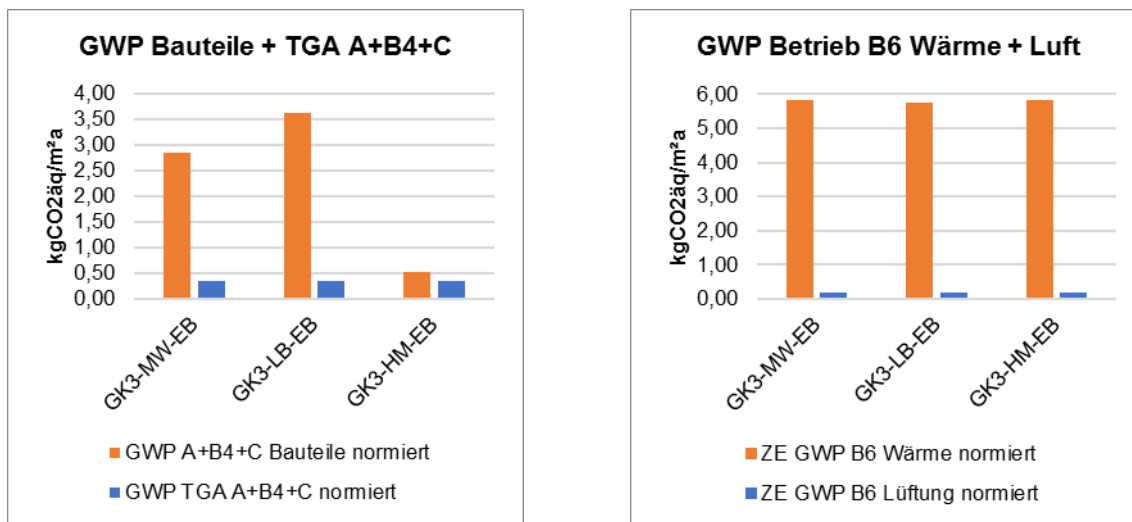
Abbildung 9: Gebäudeklasse 3 GWP Bauteile + TGA und Betrieb pro m 2 NF
