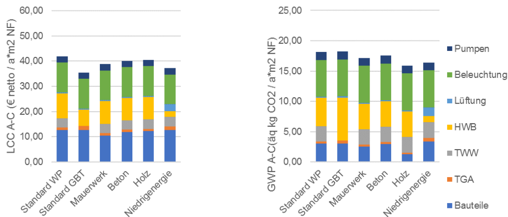
Abbildung 77 Gesamt betrachtung LCC (links) und LCA (rechts) auf Gebäudeebene GK4 (Zeile) pro m^2 NF und a
