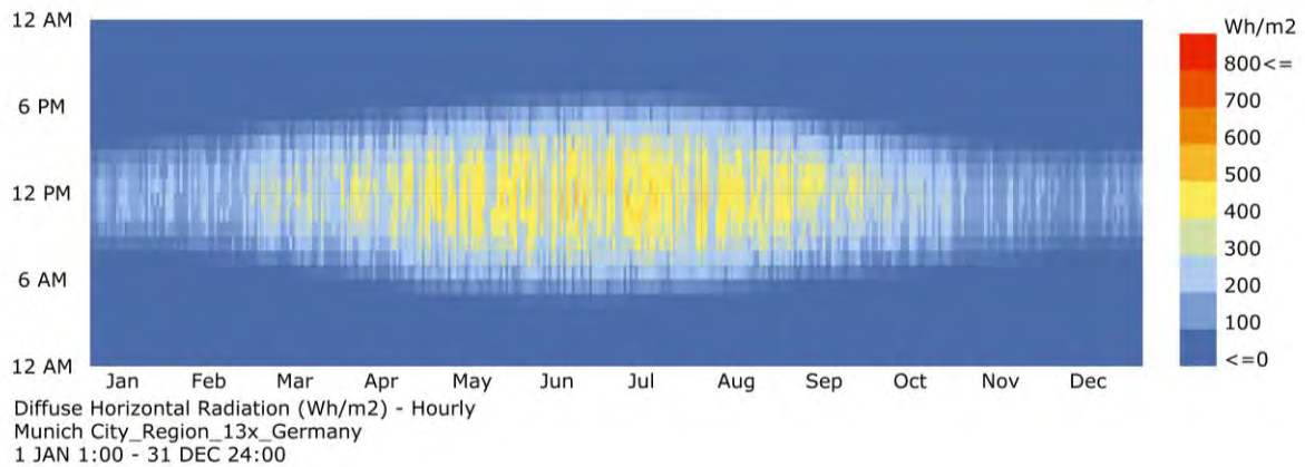
Abbildung 36: Verlauf der diffusen Horizontalstrahlung über Jahr (X-Achse) und Tag (Y-Achse)
