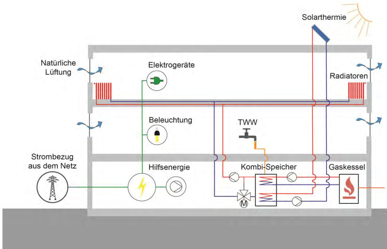
Abbildung 70: Energiekonzept EnEV-Standard
