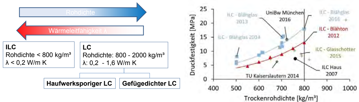
Abbildung 7: Links: Übersicht LC und ILC; Rechts: Druckfestigkeiten und Rohdichten verschiedener ILC-Zusammensetzungen aus (Schlaich and Hückler, 2017)
