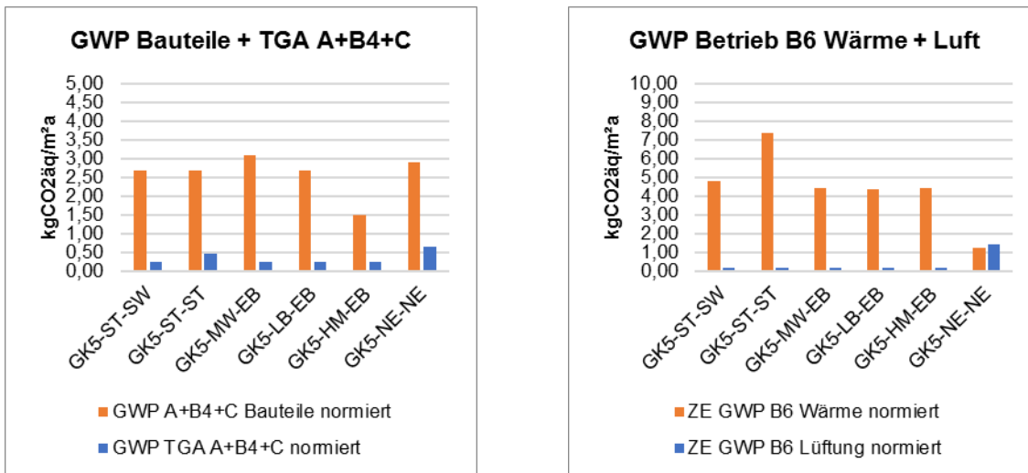
Abbildung 3: Gebäudeklasse 5 GWP Bauteile + TGA und Betrieb pro m² NF
