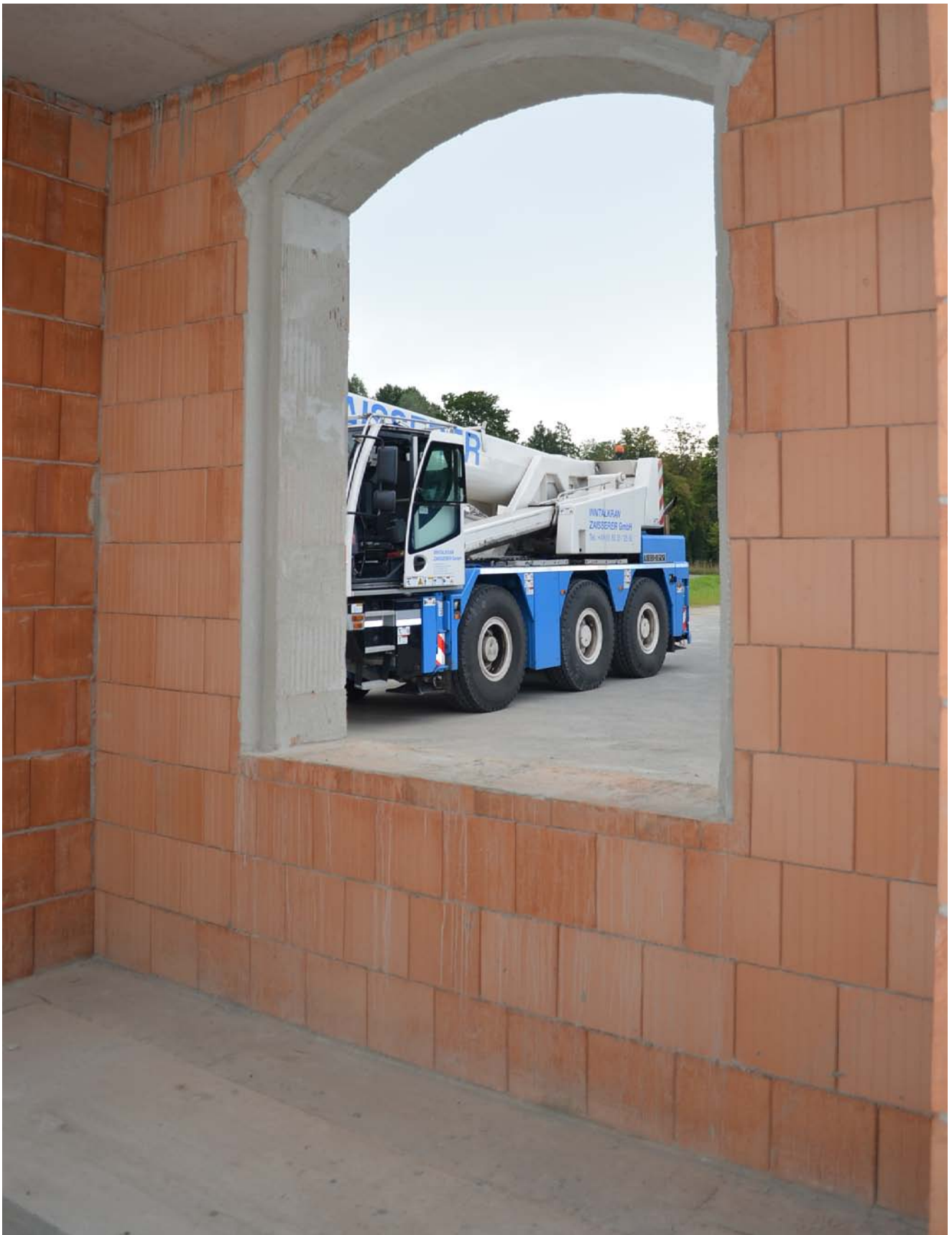
Innerer Anschlag für Fenster mit aufgebrachtem Putz-Glattstrich
