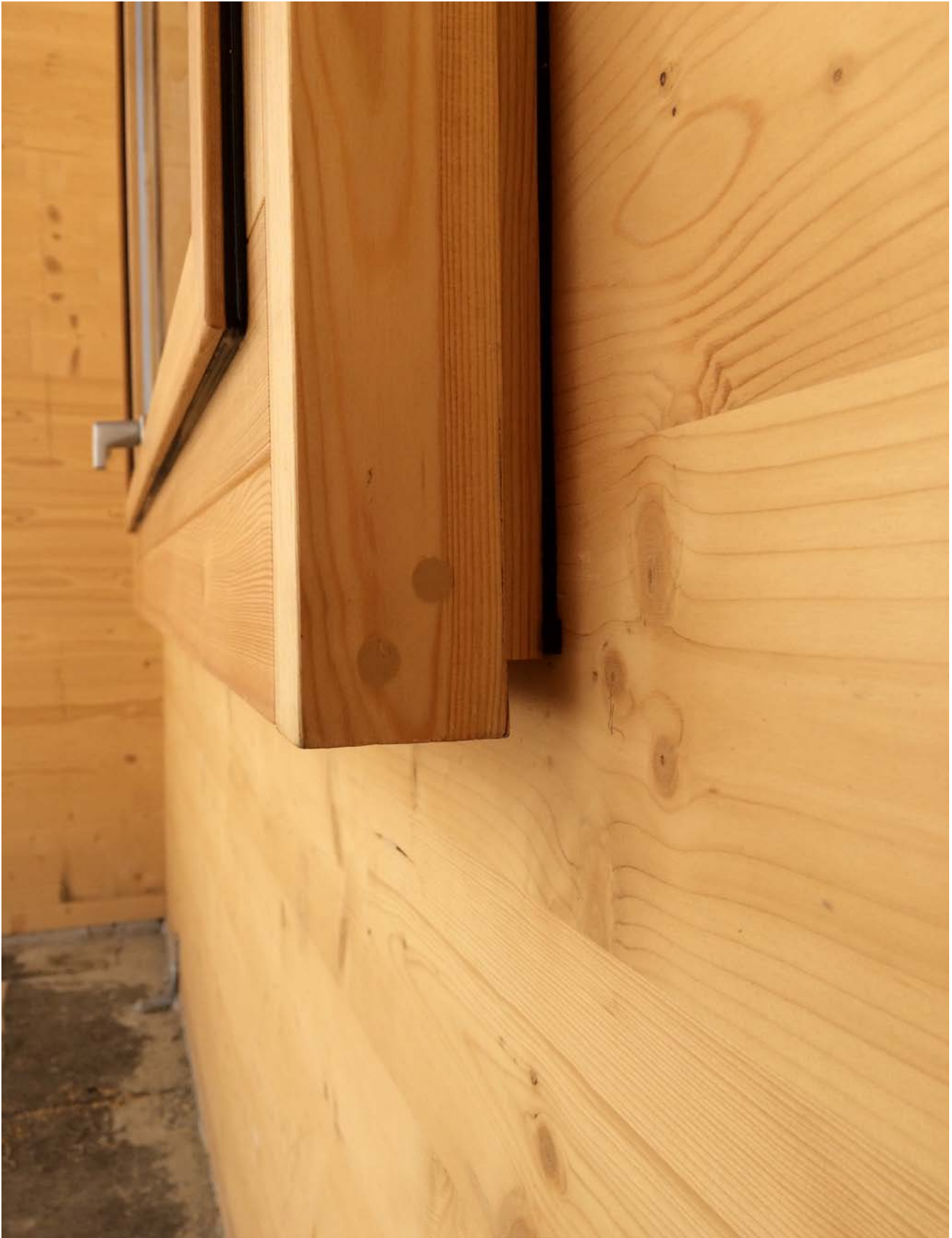
Fenster auf Innenseite der Holzmassivwand aufgesetzt und mit Quellbändern abgedichtet
