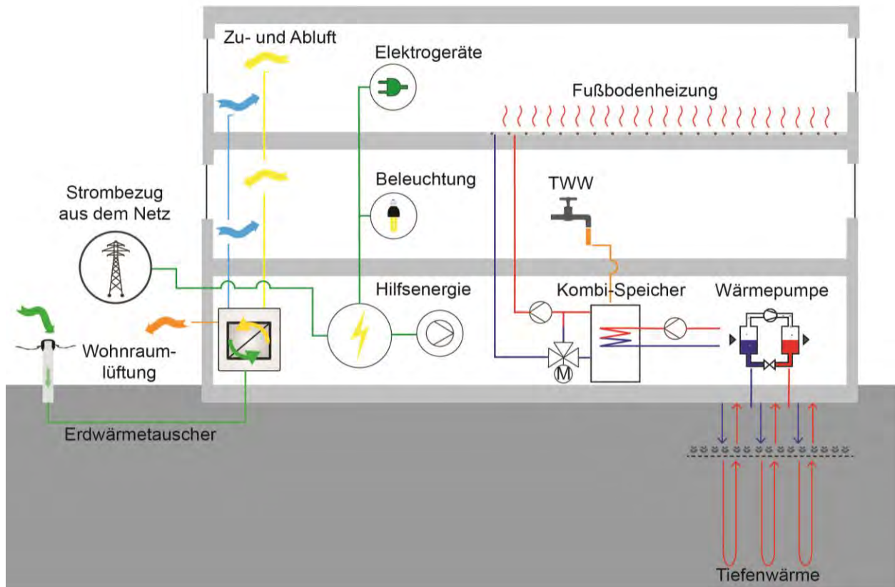
Abbildung 71: Energiekonzept Niedrigenergiestandard
