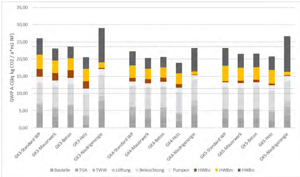
Abbildung 86: LCA zur Robustheit über den Lebenszyklus mit minimalen, normalen oder maximalen Heizwärmebedarf
