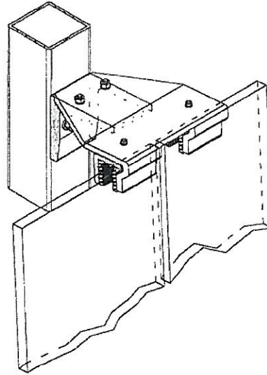
System DUO - mittlere Glasaufnahme
