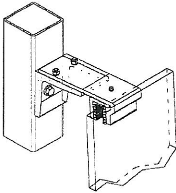
System MONO - obere Glasaufnahme
