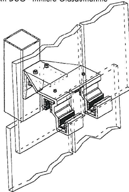
System DUO - untere Glasaufnahme
