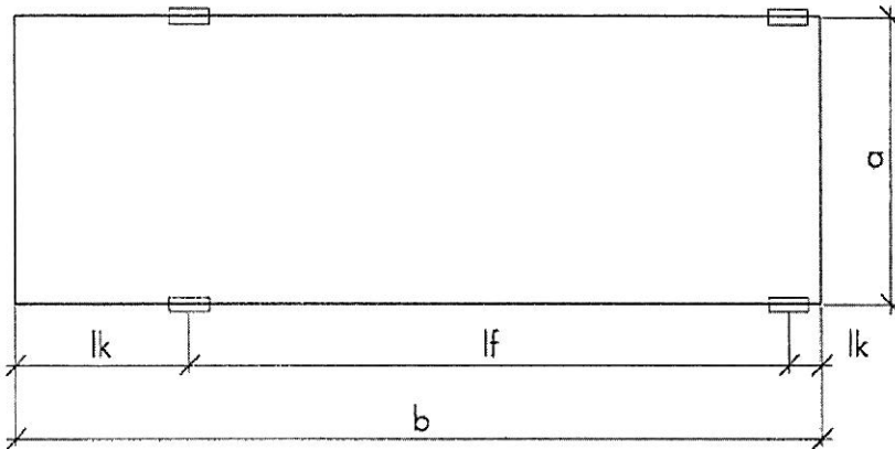
links: Halter MONO rechts: Halter DUO
