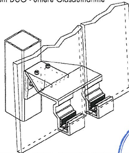
System DUO - untere Glasaufnahme
