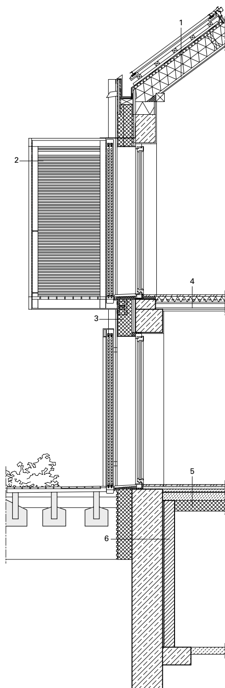
Fassadenschnitt, M 1: 50
