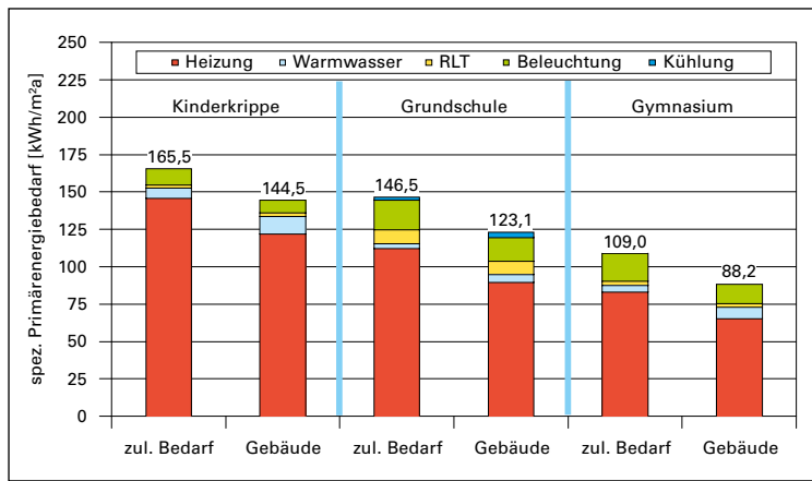
Abb. 1: Primärenergiebedarf der drei Gebäude bei Gasversorgung. Der zulässige Bedarf ist nach den bisherigen Anforderungen der EnEV 2014 berechnet, der errechnete Bedarf des Gebäudes nach LHM Standard
