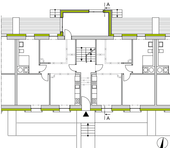
Grundriss EG, M 1:200
