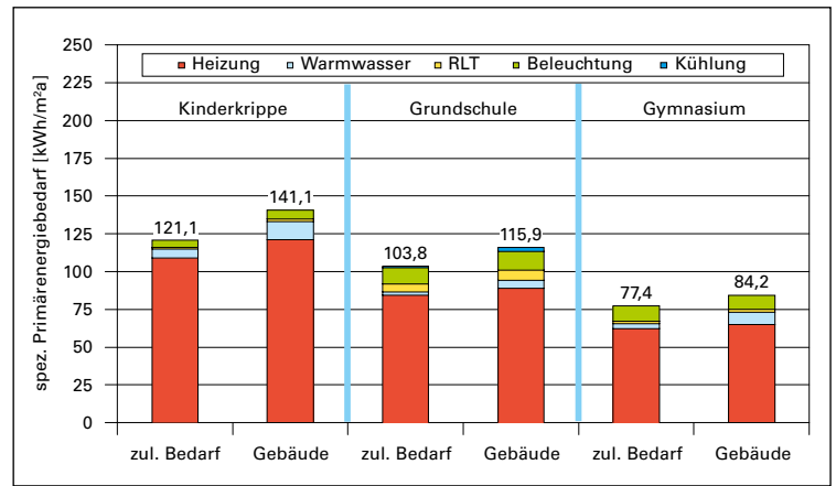
Abb. 2: Primärenergiebedarf der drei Gebäude bei Gasversorgung. Der zulässige Bedarf ist nach den ab 1.1.2016 verschärfte Anforderungen der EnEV 2014 berechnet, der errechnete Bedarf des Gebäudes nach LHM Standard
