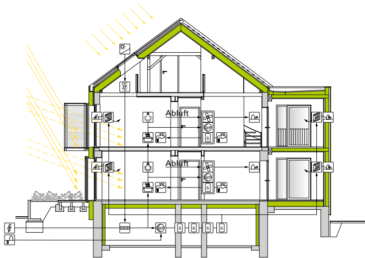
Energieschema
